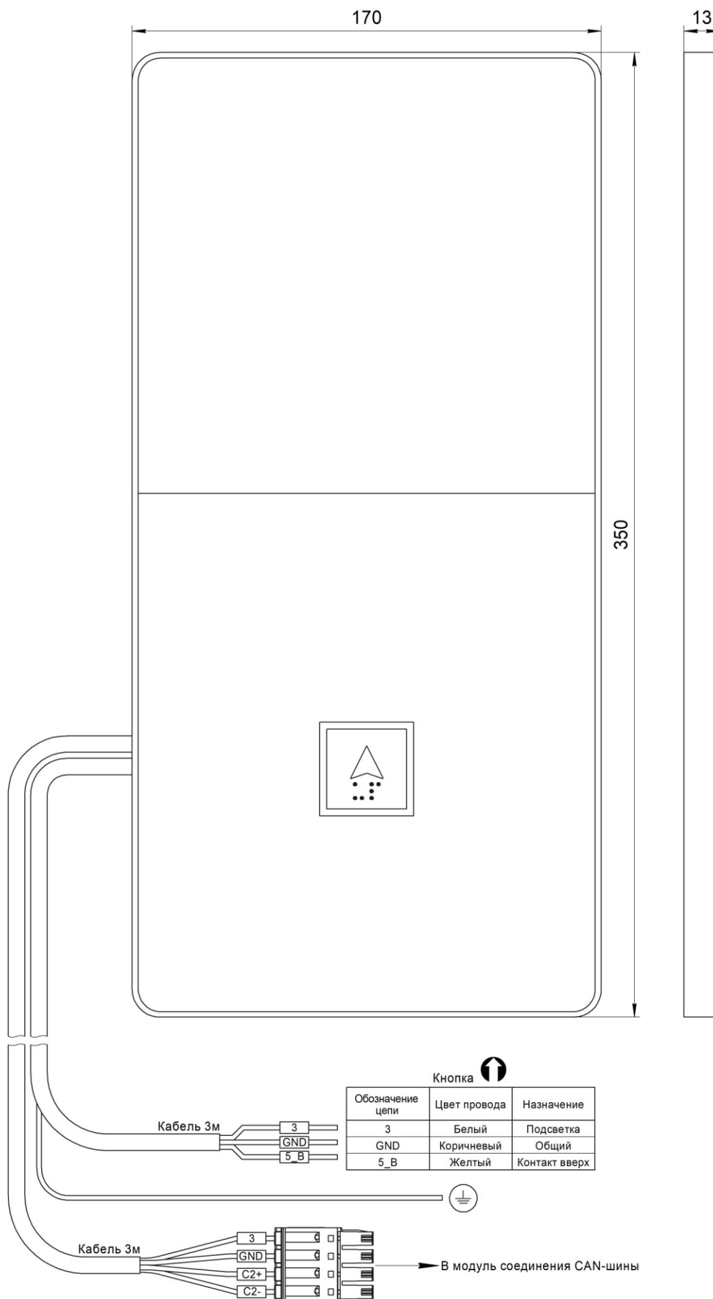
Рис.1 Внешний вид, габаритные и установочные размеры Вызывного поста МАЛАХИТ НШЕК.468381.088
